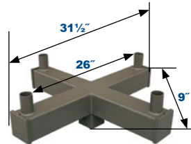
5" 90° Quad Square Vertical Tenon TS5Q180VT
